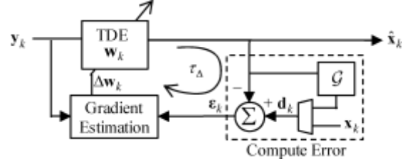
Fig. 8. Adaptive TDE.
