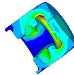
Fig. 10.1 Von mises stresses
