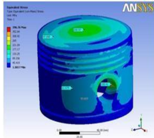
Fig. 10.2 Von mises stresses
