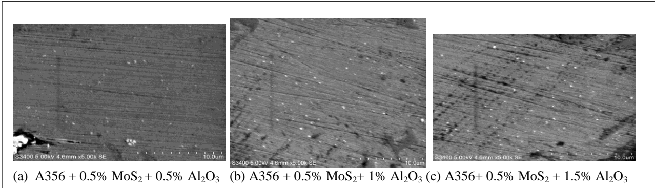
Fig 3: SEM of A356/Al 2 O 3 /MoS 2 hybrid Nano composite
